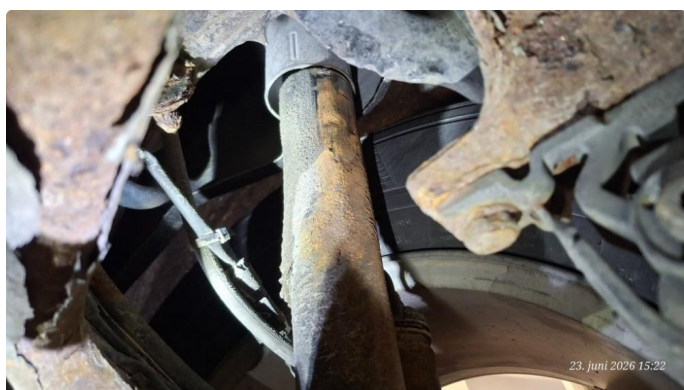
5.3 Støtdemper lekkasje
