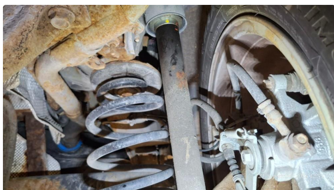
6.1 Støtdemper lekkasje
