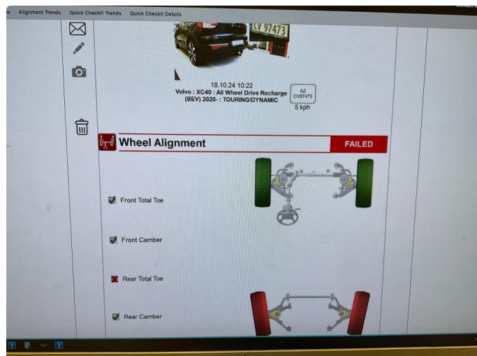
2.1 4-hjulsmåling/forstillingskontroll
