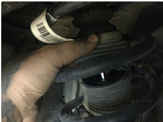
2.1 Støvmansjett defekt
