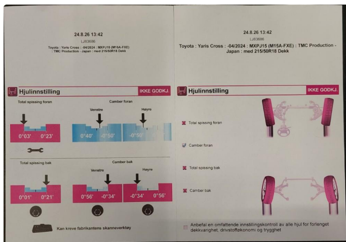
2.1 4-hjulsmåling/forstillingskontroll
