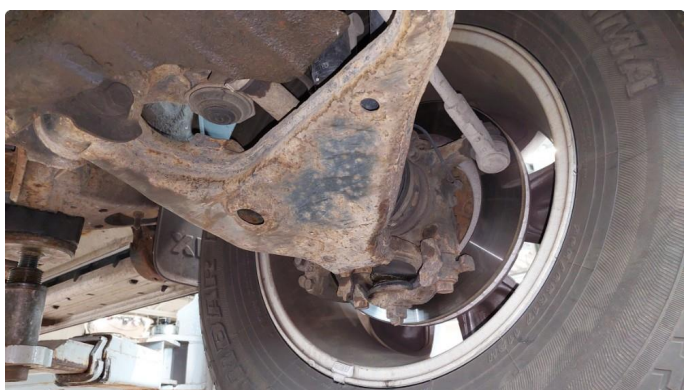
4.2 Mansjett bærekule defekt
