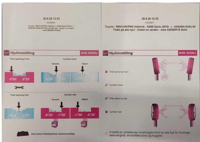
2.1 4-hjulsmåling/forstillingskontroll
