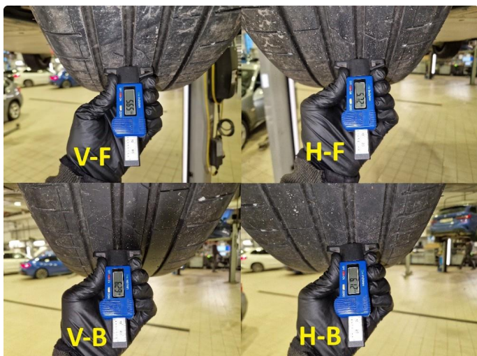
1.1 Dekkdybdemåling sommerdekk utført 08.07.2026 på km : 21.469
