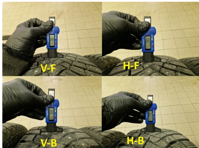
1.2 Dekkdybdemåling vinterdekk utført 08.07.2026 på km : 21.469
