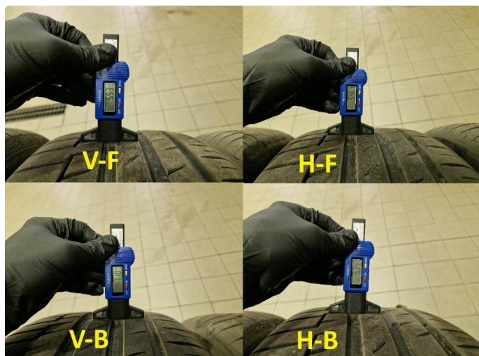
1.1 Dekkdybdemåling sommerdekk utført 16.06.2026 på km : 33.942.
