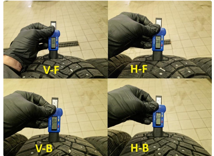
1.2 Dekkdybdemåling vinterdekk utført 07.08.2026 på km : 123.158.
