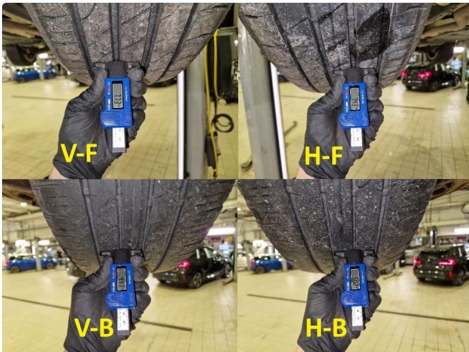
1.1 Dekkdybdemåling sommerdekk utført 07.08.2026 på km : 123.158.
