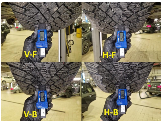
1.4 Dekkdybdemåling vinterdekk utført 19.03.2026 på km : 114.475.
