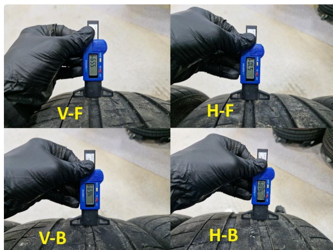
1.3 Dekkdybdemåling sommerdekk utført 19.03.2026 på km : 114.475.
