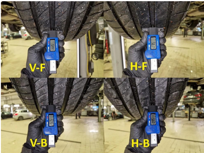
1.1 Dekkdybdemåling sommerdekk utført 27.05.2026 på km : 174.159
