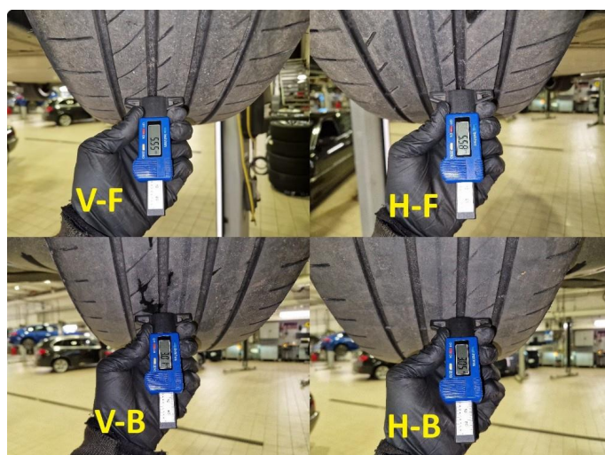
1.3 Dekkdybdemåling sommerdekk utført 18.08.2026 på km : 84.778. 2 nye bak dekk på satt etter takst.
