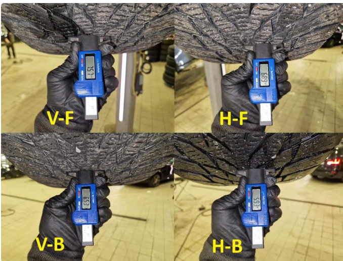
1.3 Mønsterdybde vinterdekk målt ved takst 30.04.2025, 77.429km.
