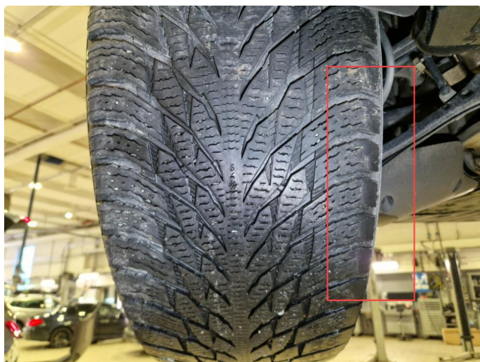
1.6 Noe skjeivslitasje innside vinterdekk h+v bak . ( Normal bruksslitasje )
