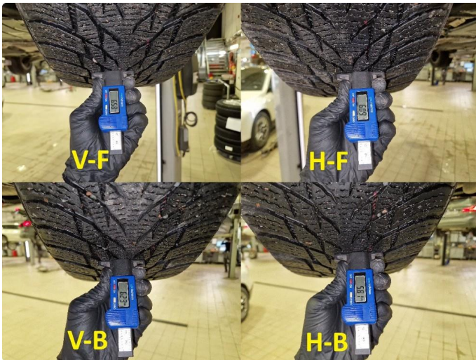
1.1 Dekkdybdemåling vinterdekk utført 05.11.2025 på km : 51.908
