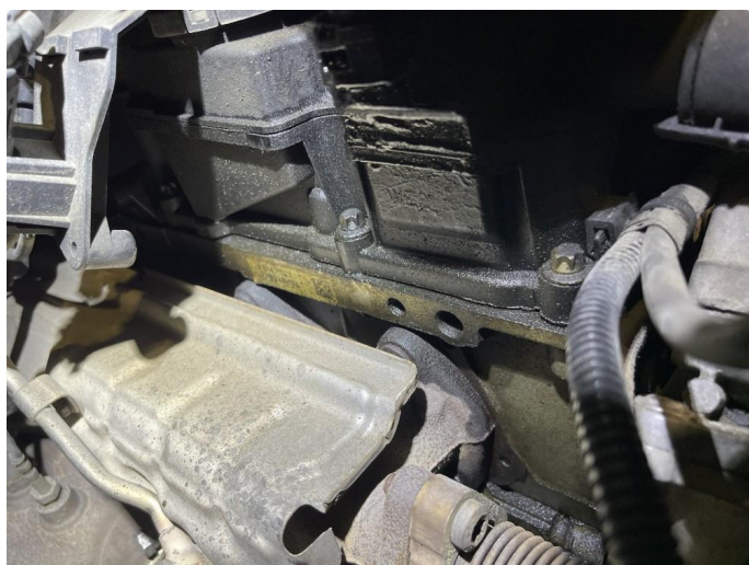
4.1 Lekkasje/svetting fra toppdeksel.
