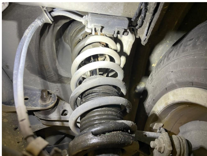
5.2 Støvmansjett defekt
