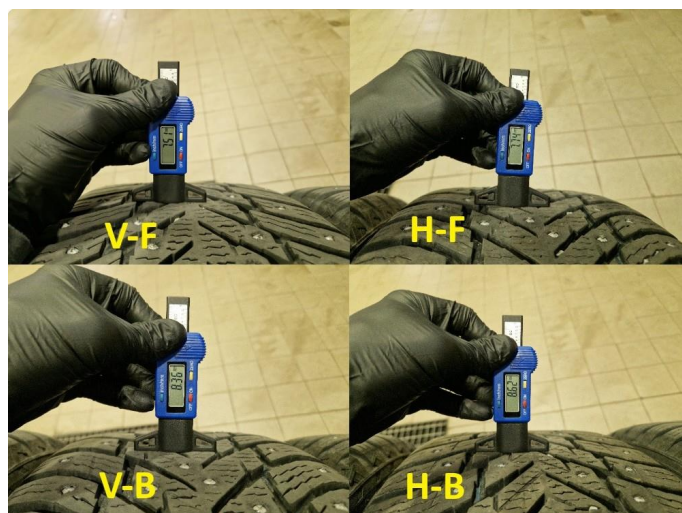
1.3 Dekkdybdmåling vinterdekk utført 26.06.2026 på km : 45.231.
