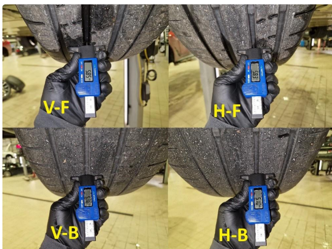
1.2 Dekkdybdmåling sommerdekk utført 26.06.2026 på km : 45.231.
