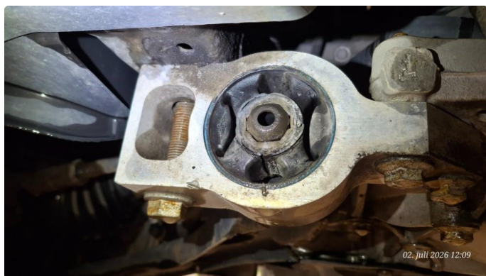
3.1 Slitt bæreforfing
