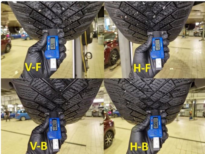
1.1 Dekkdybdemåling vinterdekk utført 24.08.2026 på km : 106.054.
