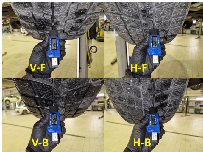
1.2 Dekkdybdemåling vinterdekk utført 30.03.2026 på km : 120.545.
