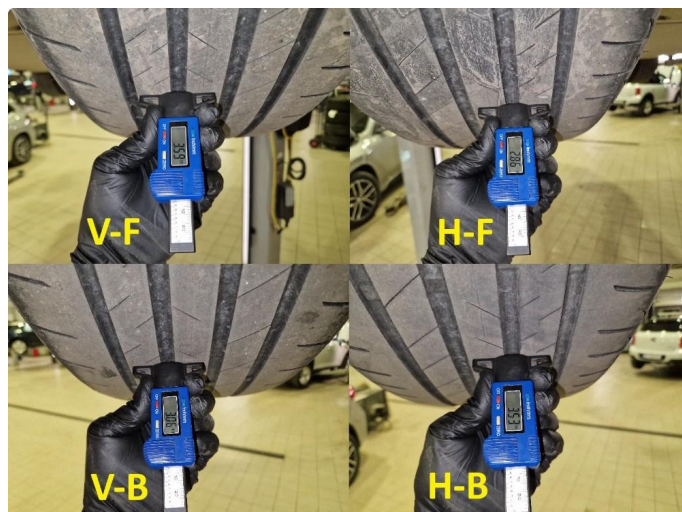
1.2 Dekkdybdemåling sommerdekk utført 11.05.2026 på km : 35.741
