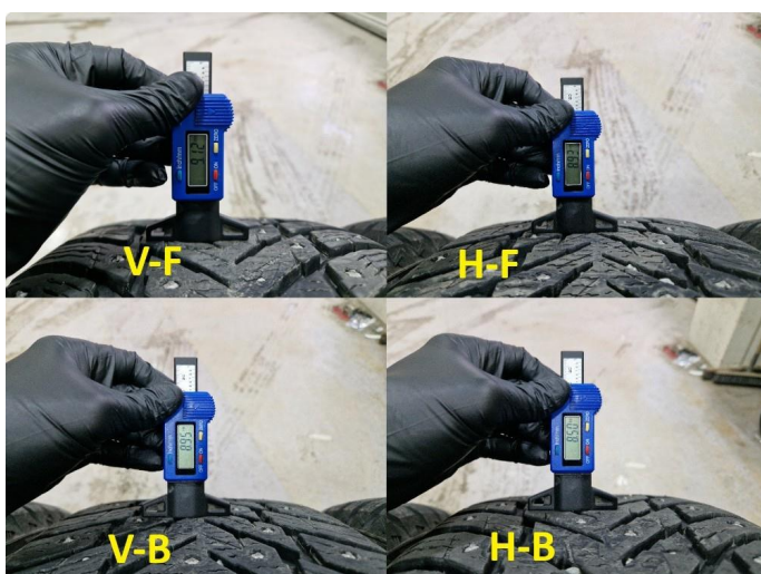
1.3 Dekkdybdemåling vinterdekk utført 11.05.2026 på km : 35.741
