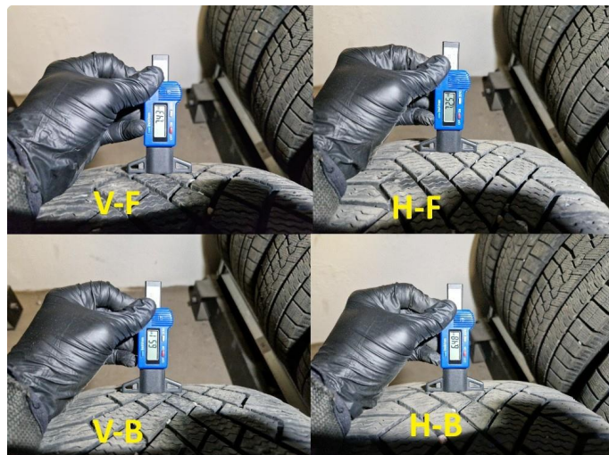
1.2 Dekkdybdemåling vinterdekk utført 30.09.2026 på km : 45.294.
