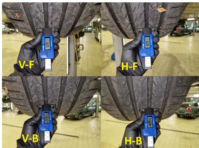
1.1 Dekkdybdemåling sommerdekk utført 30.09.2026 på km : 45.294.
