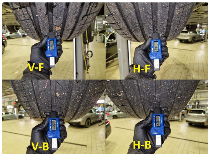
1.1 Dekkdybdemåling sommerdekk utført 21.09.2026 på km : 9.405.
