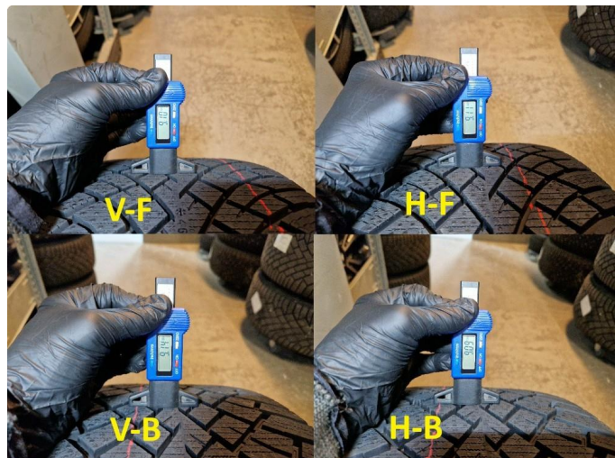
1.2 Dekkdybdemåling vinterdekk utført 21.09.2026 på km : 9.405.
