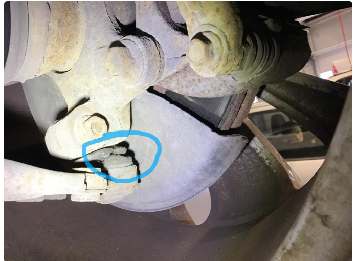
2.1 Skiftet nedre bærekule foran begge sider.
