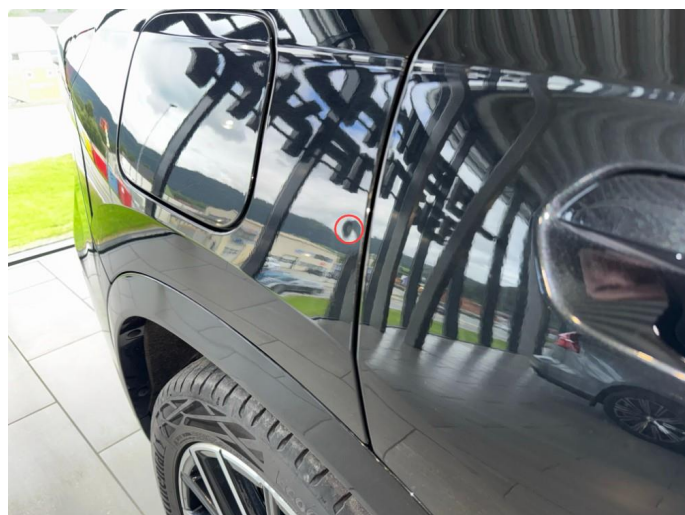
1.3 PDR-bulk
