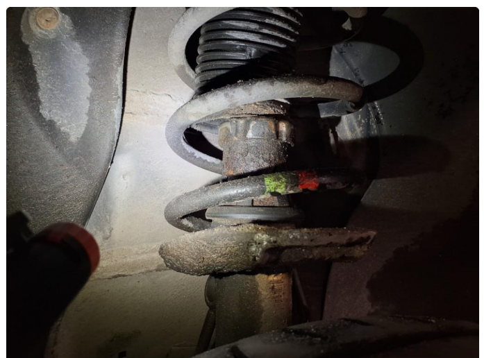
3.1 Støtdemper lekkasje
