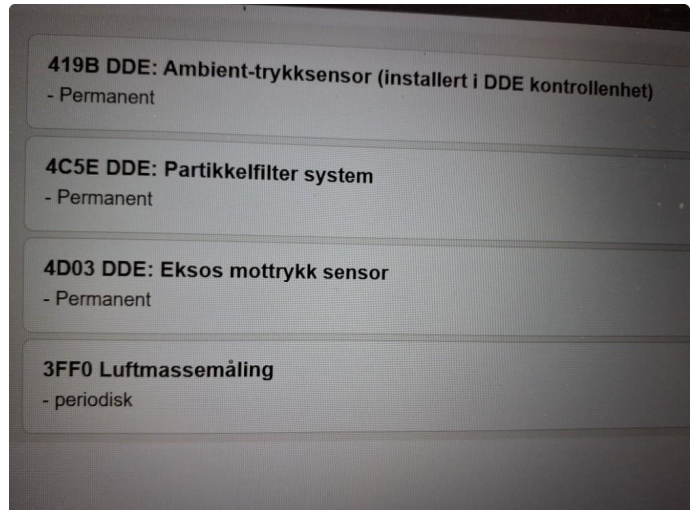
2.2 Flere permanente feillager, blant annet på partikkelfilter, Må videre feilsøkes.
