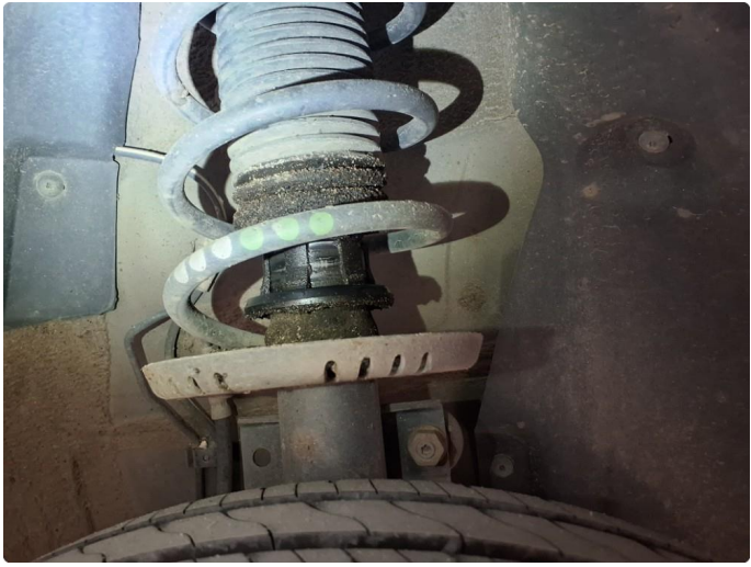
3.1 Støtdemper lekkasje , begge foran
